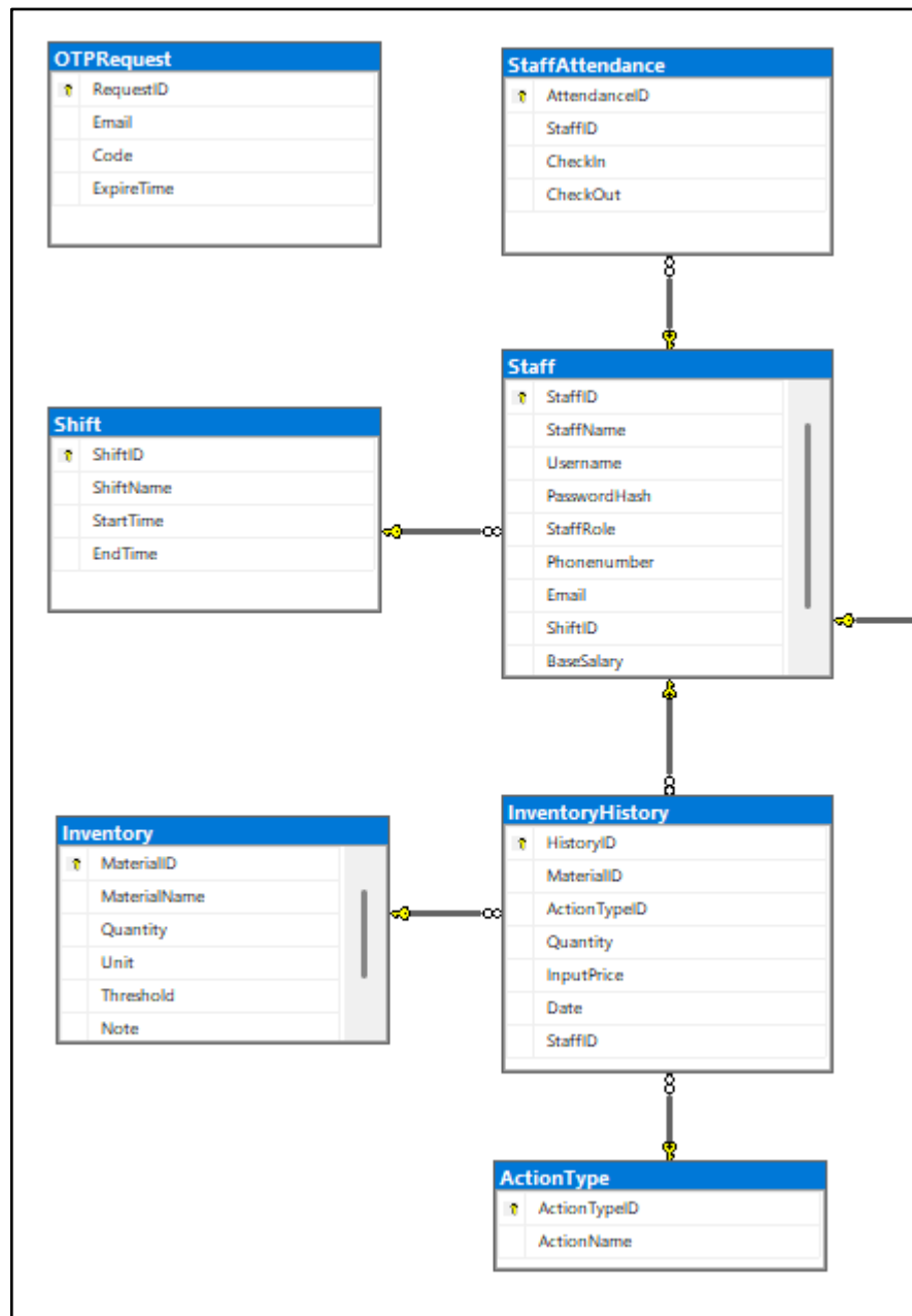
Hình 3. Các bảng phục vụ chức năng đăng nhập, phân quyền, quản lý nhân viên, quản lý ca làm việc và quản lý kho hàng.
