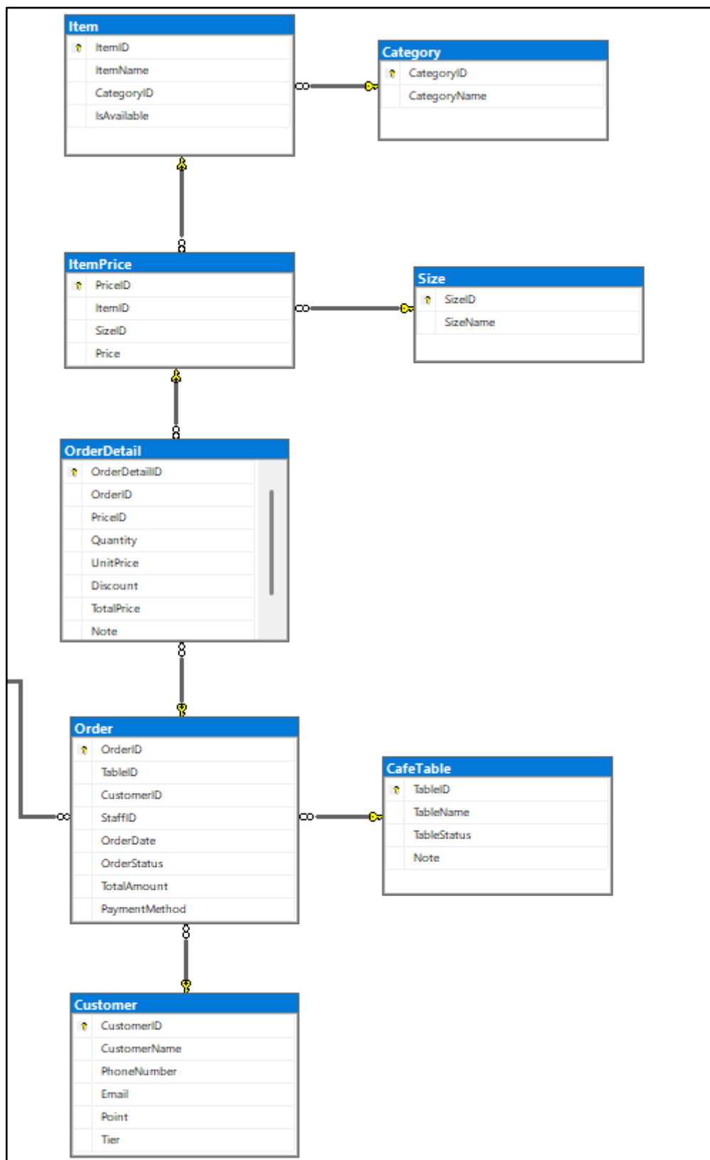
Hình 2. Các bảng phục vụ chức năng bán hàng, quản lý bàn, quản lý hóa đơn, quản lý menu, quản lý khách hàng
