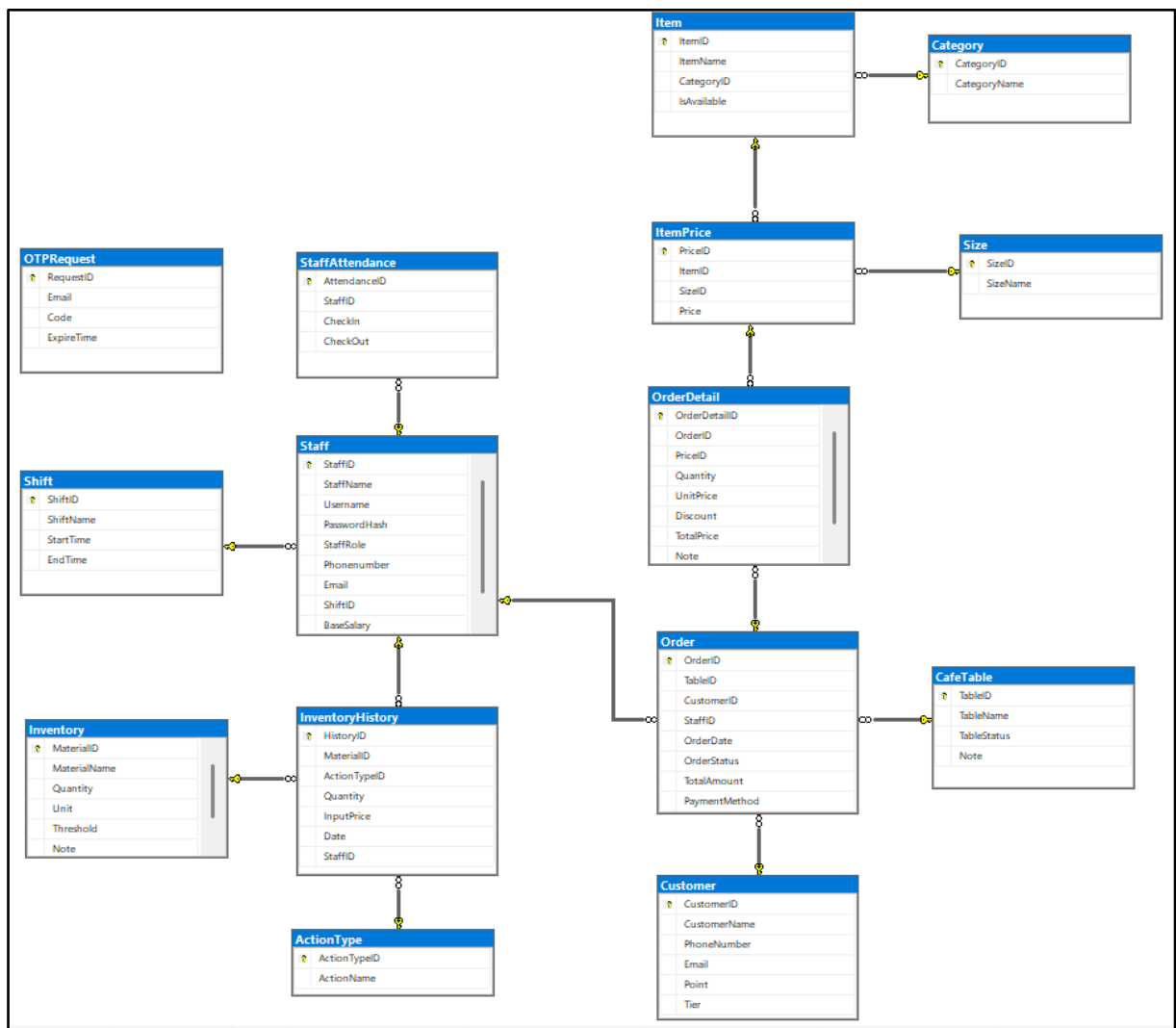
Hình 1. Database diagram tổng quát
